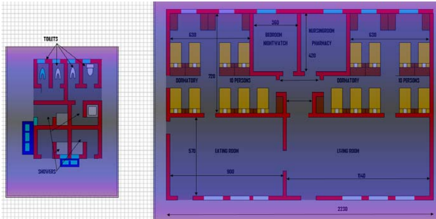
Plan des deux bâtiments pour les dortoirs, salle à manger, toilettes et douches
