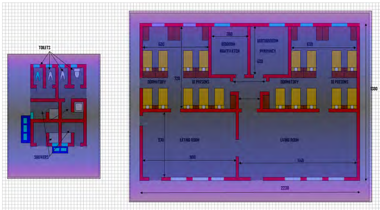
Plan des deux bâtiments pour les dortoirs, salle à manger, toilettes et douches
